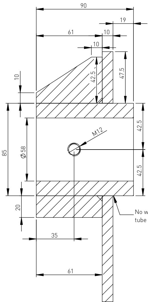
SECTION A-A
